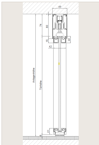
Deckenmontage 1 lfg. auf Putz
