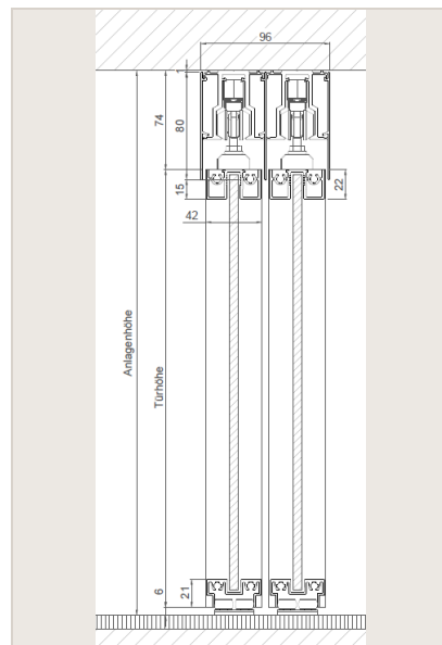
Deckenmontage 2 lfg. auf Putz
