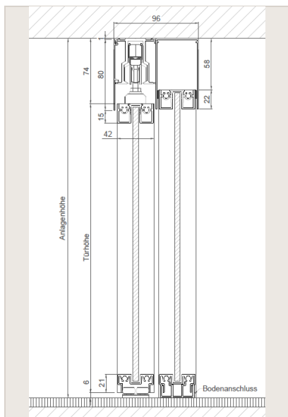
Deckenmontage mit Fixteil
