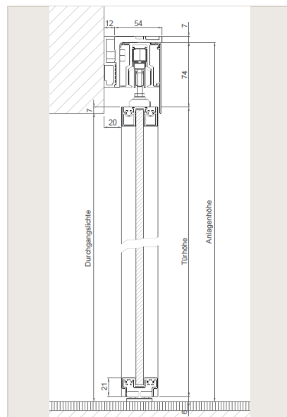
Wandmontage 1 lfg. mit Wanddistanzprofil
