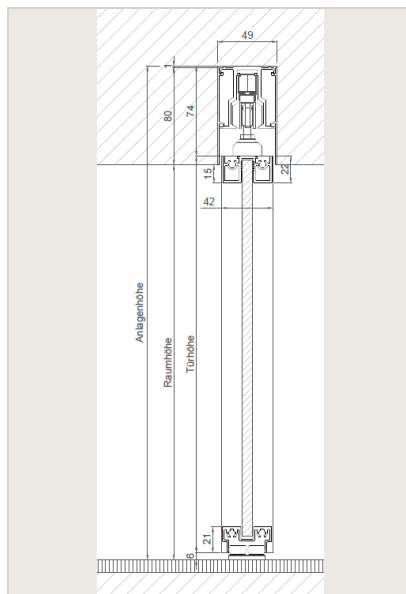
Deckenmontage 1 lfg. eingelassen
