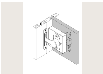
Schloss Serie 1200 Druckriegelschloss zum Versperren zweier hintereinanderstehenden Türen
