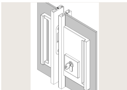
Schloss Serie 1200 Drehriegelschloss zum Versperren zweier nebeneinanderstehender Türen
