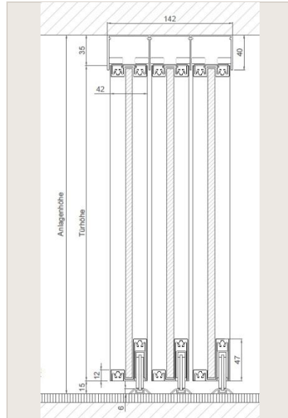
Bodenschiene 3 lfg. aufgelegt
