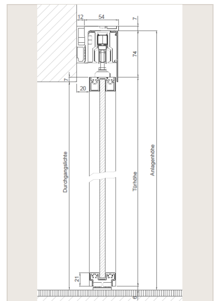
Wandmontage 1 lfg. mit Wanddistanzprofil
