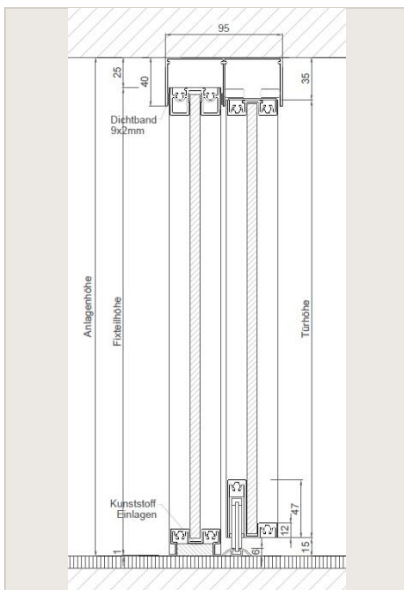
Tür und Fixteil
