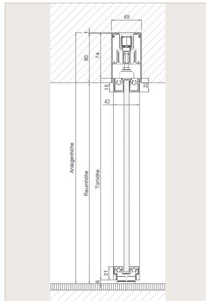
Deckenmontage 1 lfg. eingelassen
