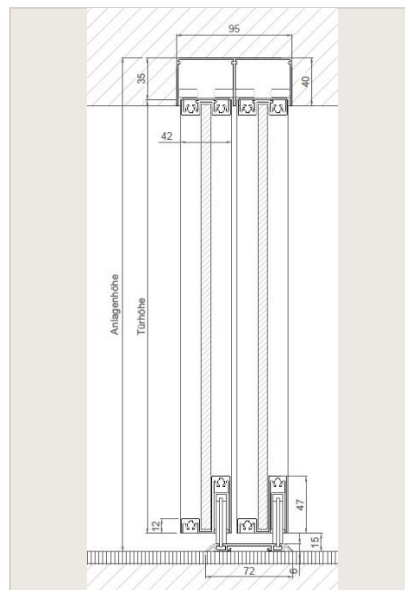
Deckenschiene eingelassen
