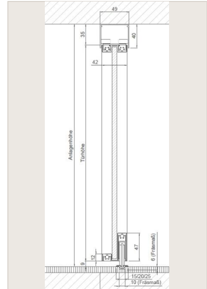
Bodenschiene 1 lfg. zum Einfräsen
