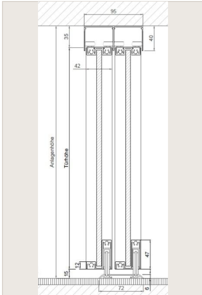
Bodenschiene 2 lfg. aufgelegt
