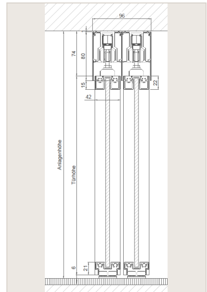
Deckenmontage 2 lfg. auf Putz
