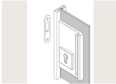
Schloss Serie 1200 Drehriegelschloss zum Versperren einer Tür direkt in die Wand
