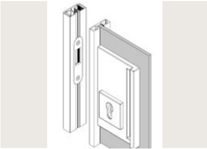
Schloss Serie 1200 Drehriegelschloss zum Versperren einer Tür in den Wandanschluss
