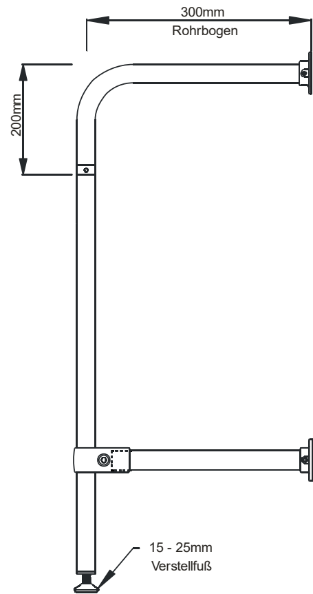
Abb. 3_Montage vom Boden zur Wand mit Rohrbogen und Maueranschluss zur Wand zur zusätzlichen Stabilisierung
