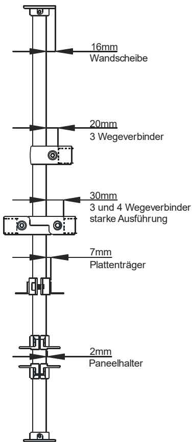
Abb.1_Abzugsmaße Chromsystem Montage vom Boden zur Decke mit Wandscheiben, kein Verstellbereich
