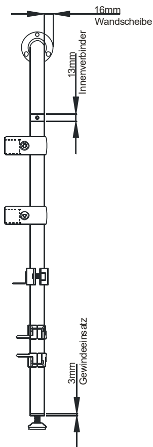
Abb. 2_Montage vom Boden zur Wand mit Verstellfuß Verstellbereich 15-25mm Anschluss zur Wand mit Rohrbogen
