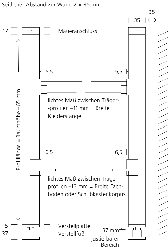
Abb. 2 Abzugsmaße Uno
