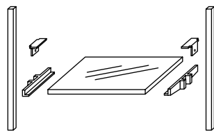
Abb. 2b Pro Glasfachboden: 2 Glasfachbodenhalter und 2 L-Träger
