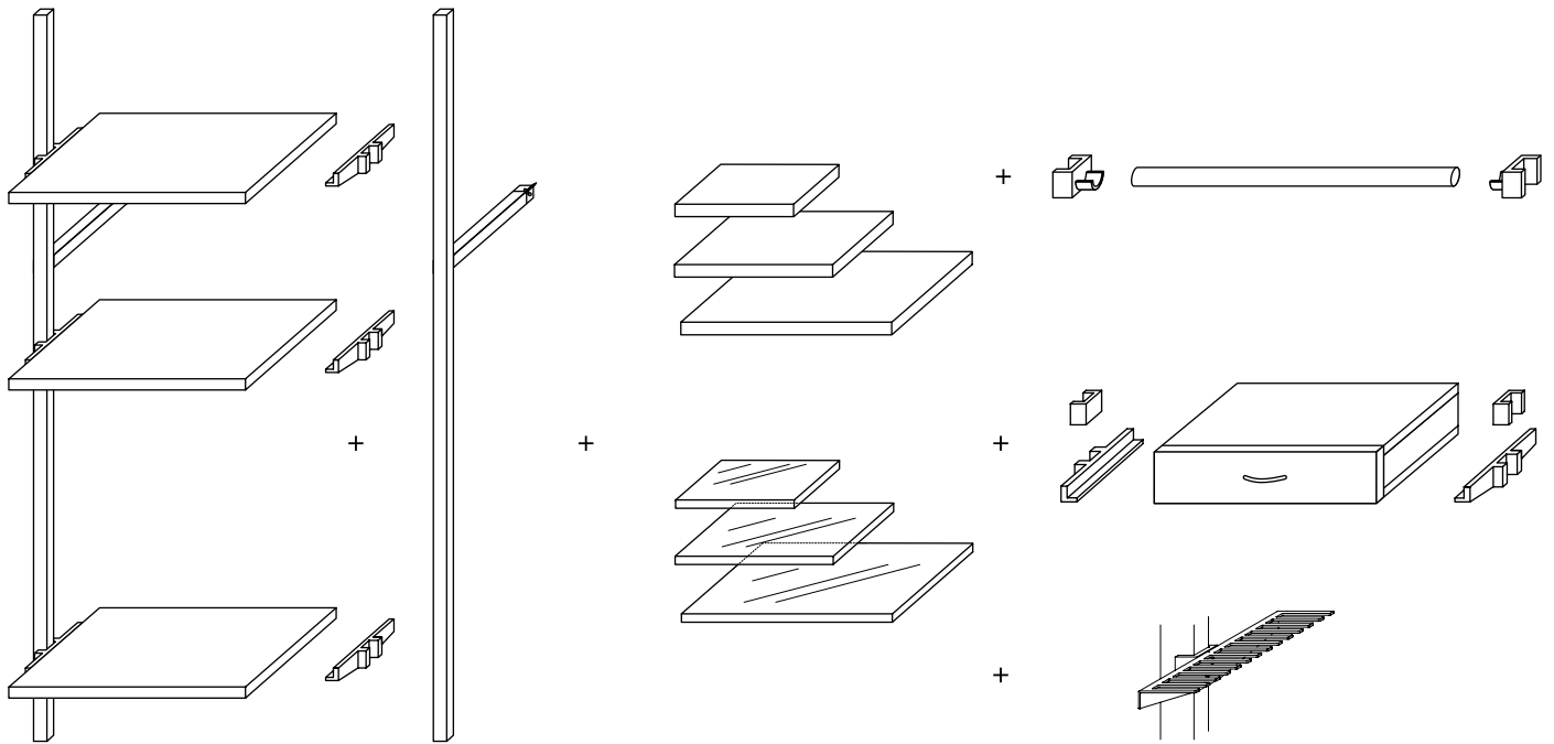
Abb. 1 Beispielelement mit rechtem Trägerprofil, Fachböden, Kleiderstange, Schubkastenkorpus und weiteren Accessoires (inkl. benötigter Verbindungselemente)
