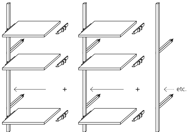
Abb. 1 zwei Beispiэлеlemente mit rechtem Trägerprofil
