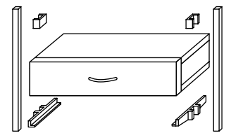
Abb. 2d Pro Schubkastenkorpus: 2 L-Träger und 2 Universalträger
