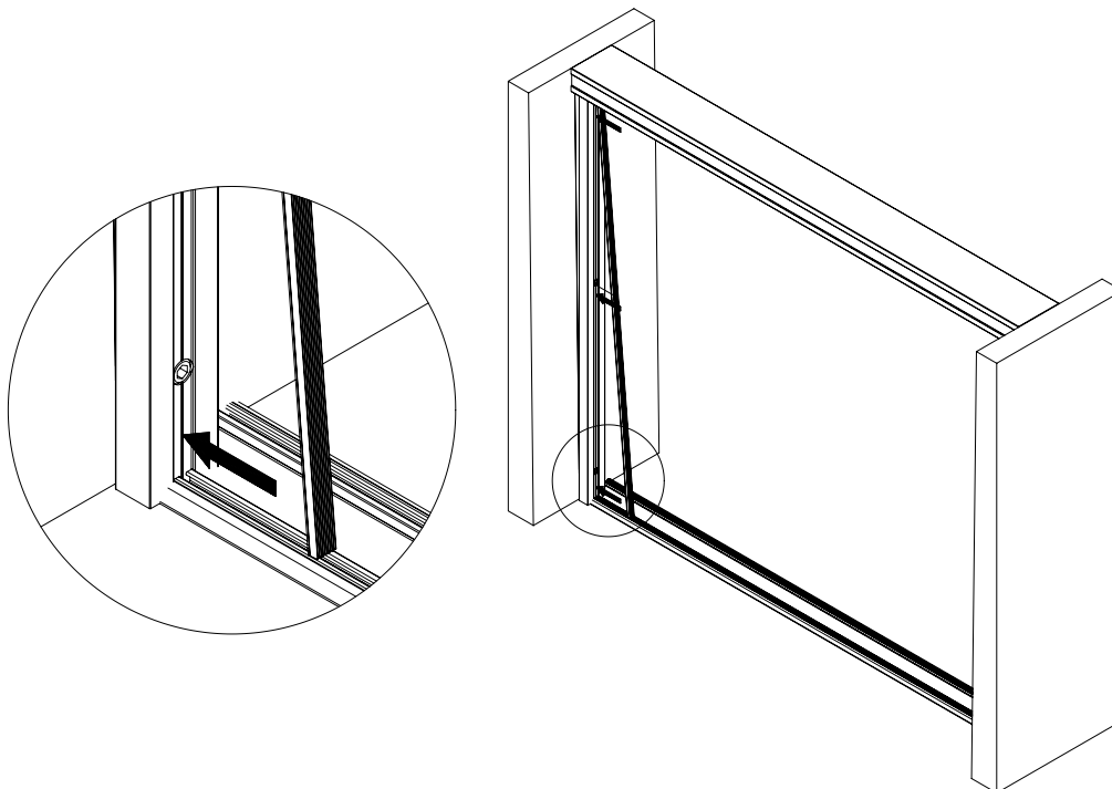
5_ Dichtungsbürste aufkleben
