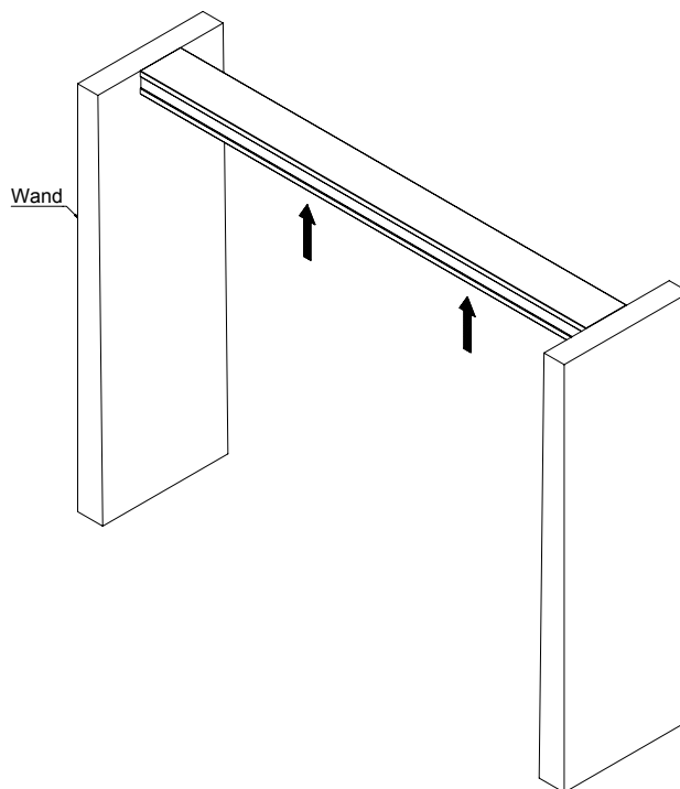
1_ Deckenschiene ausrichten und befestigen
